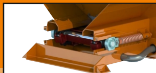
Цельнометаллический вал привода транспортера на самоцентрирующихся подшипниках качения
