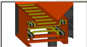
Цепной транспортер со съёмными полосовыми скребками
